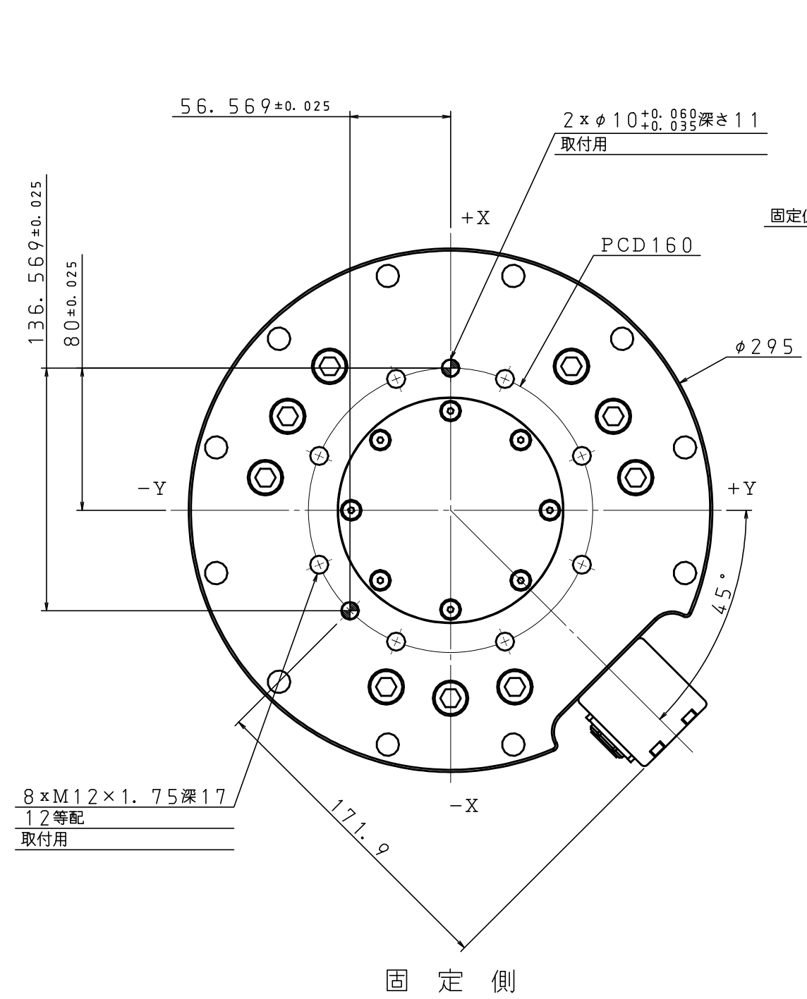
IP60 (防塵) 仕様の変換器
