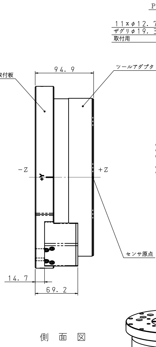
IP60 (防塵) 仕様の変換器
